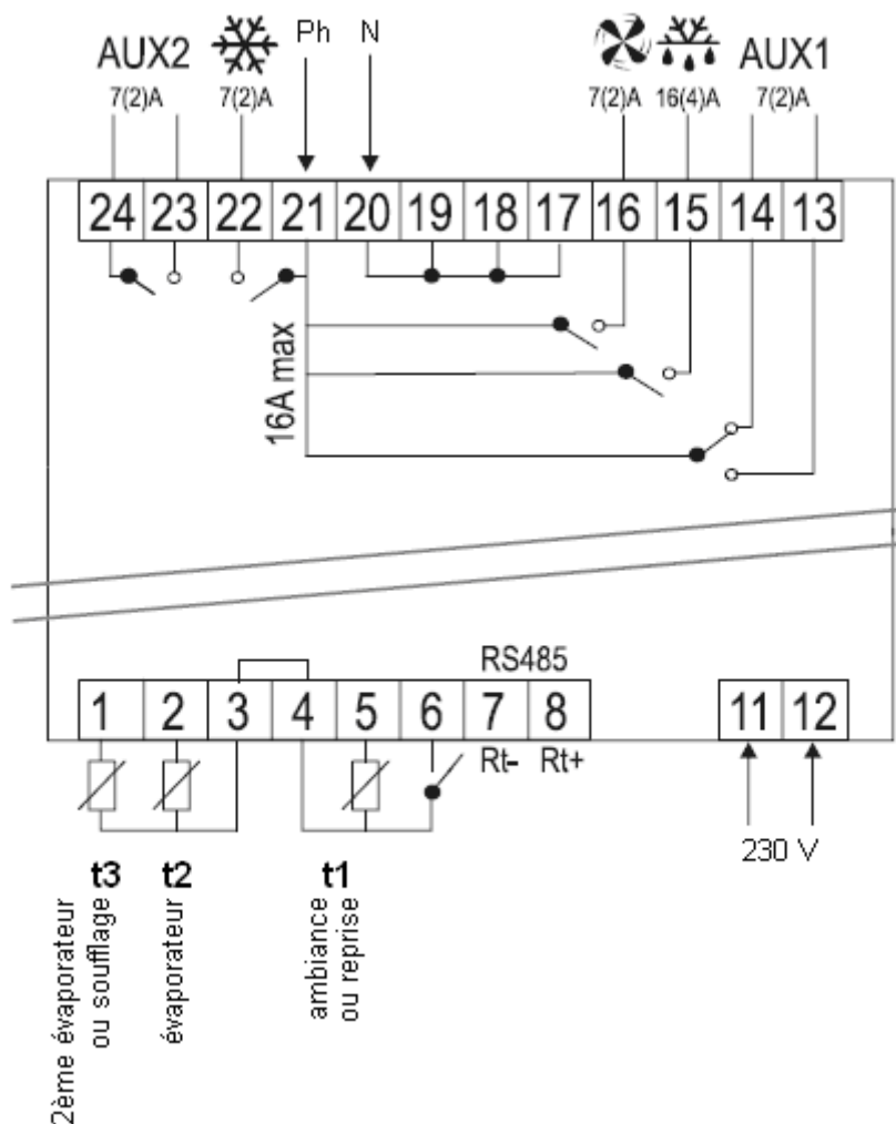
Figure 6 : Schéma de câblage
