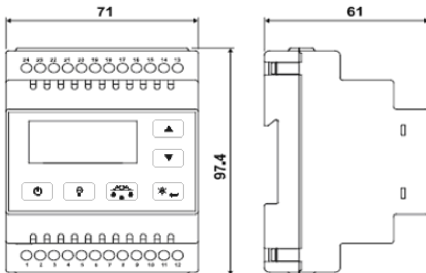
Figure 5 : Dimensions du MR55
